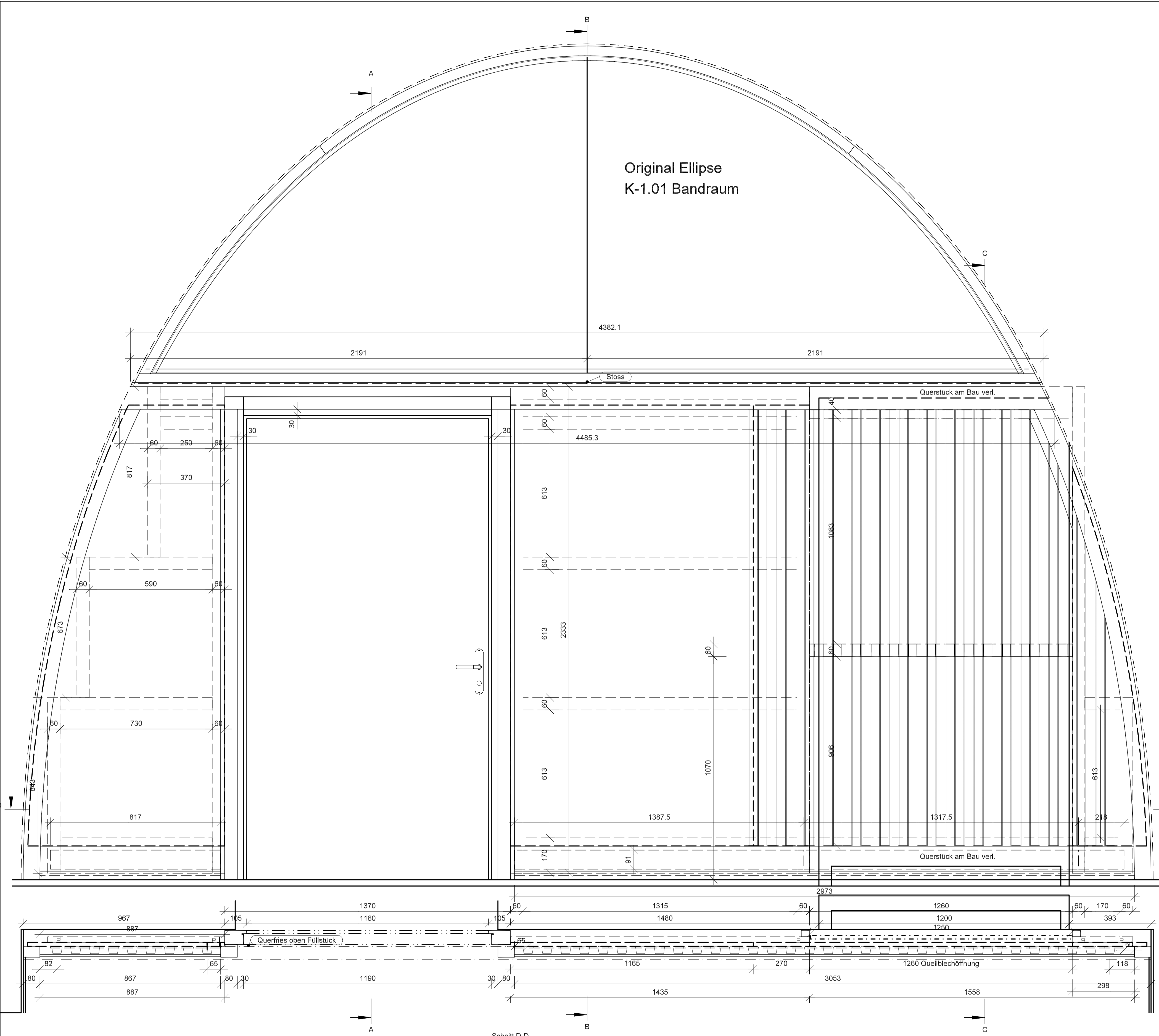
Schnitt D-D
